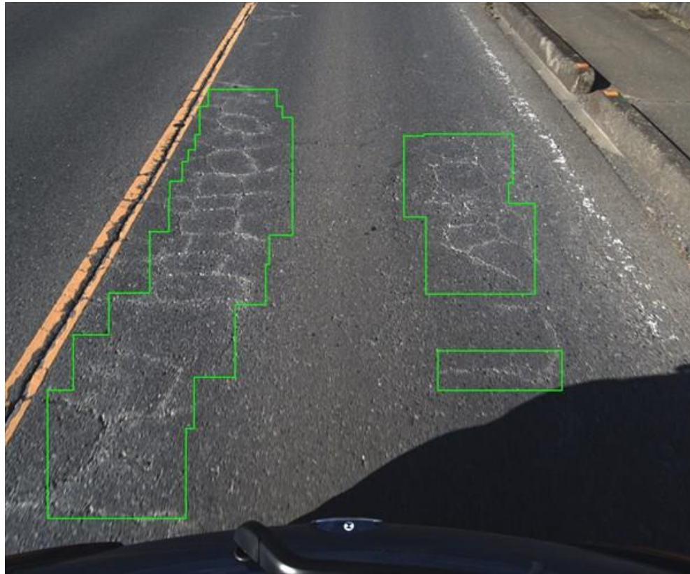
AIによるひび割れ範囲(緑枠)
