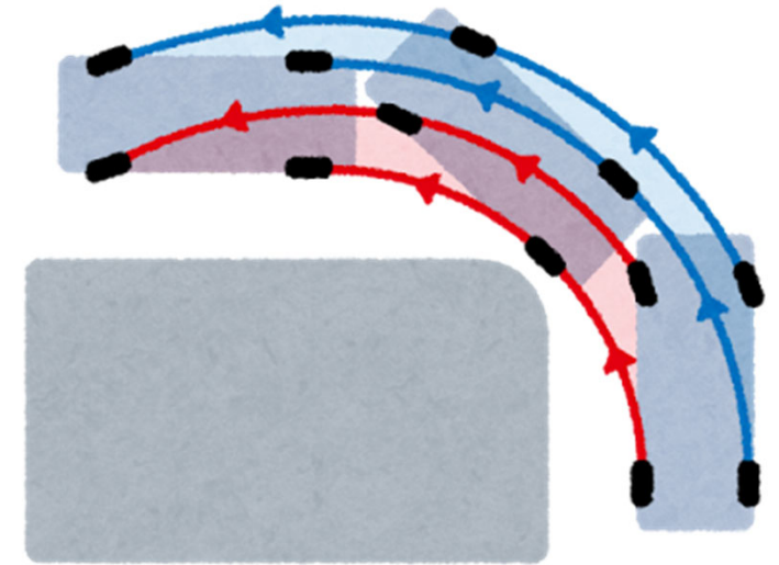
大型車両の 軌跡シミュレーション
