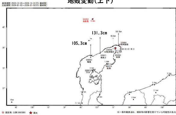
令和6年能登半島地震(1月1日 M7.6)前後の観測データ(暫定) (第5報)(第5報は2月15日発表) 地殻変動(上下) 地殻変動(水平)
