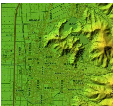
色別標高図
