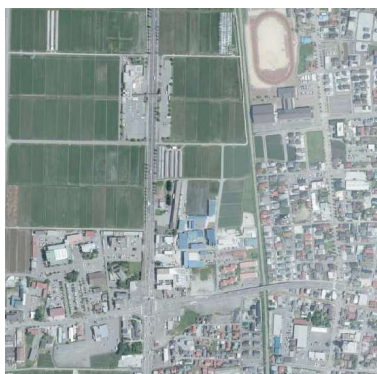
空中写真
