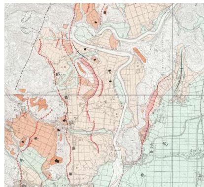
活断層図
