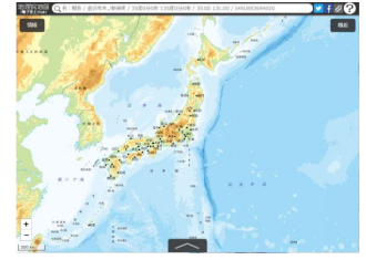
地理院地図
