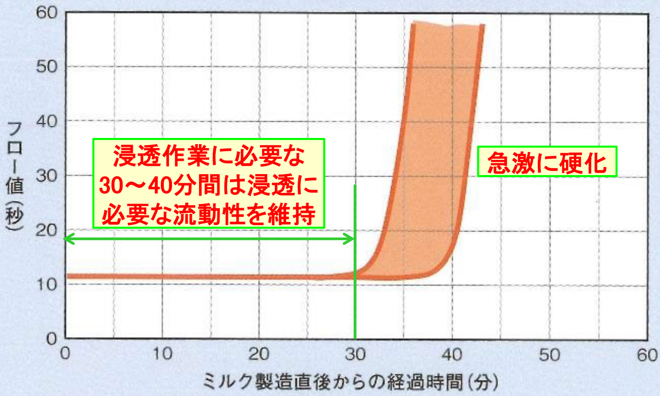
ダイヤツイン高強度ミルクの流動性
