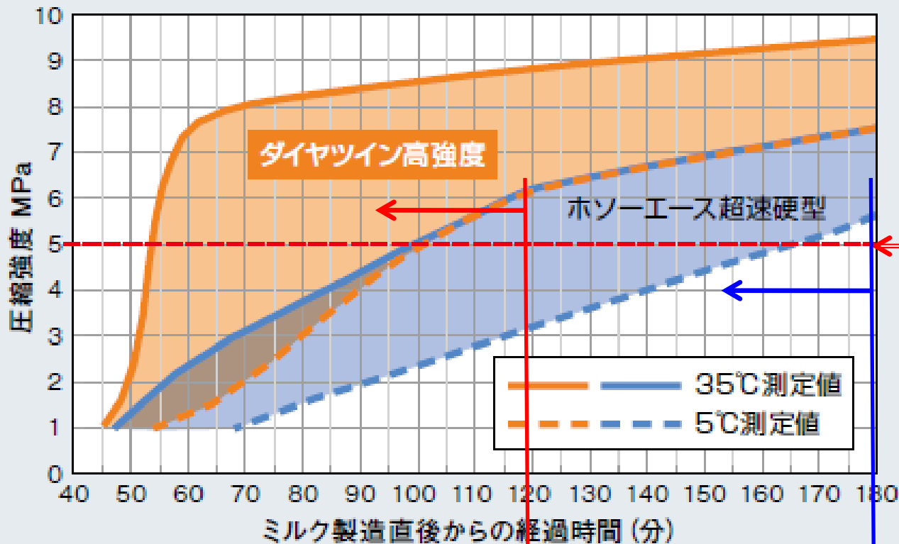
3時間までの強度発現の比較
